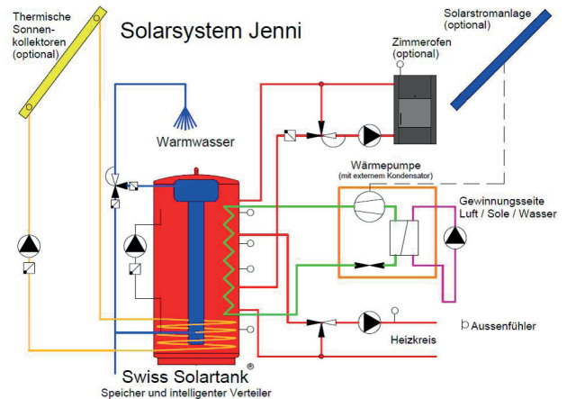
Prinzip der Anlage mit Optionen
